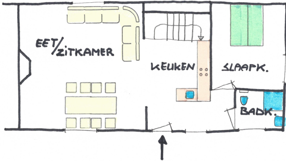
BEGANE GROND
